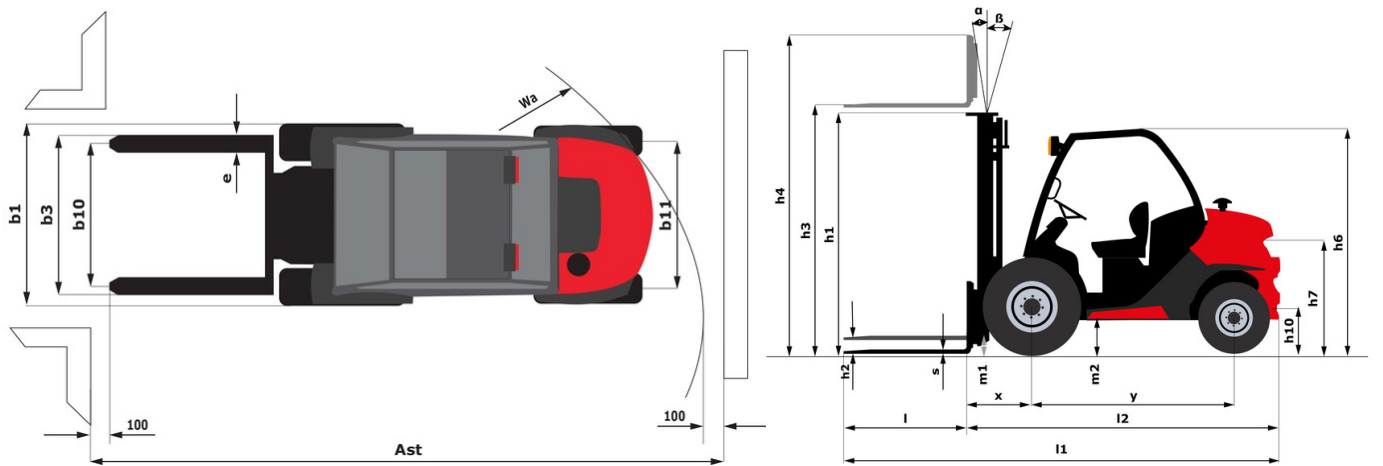
MC 25-4 ST5 - Tekening met afmetingen
